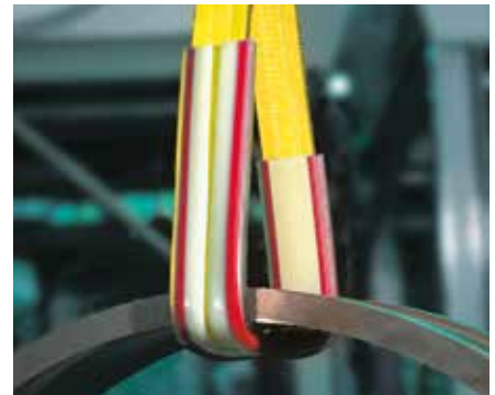
LASH+LIFT-Schutzschlauch CLIP-SC Schnittfeste secutex-Beschichtung, durch einseitige Öffnung leicht nachrüstbar.
