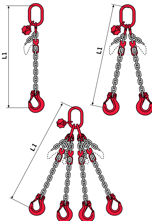
Abbildung: Verkürzungsklaue statt Verkürzungshaken gegen Mehrpreis!
